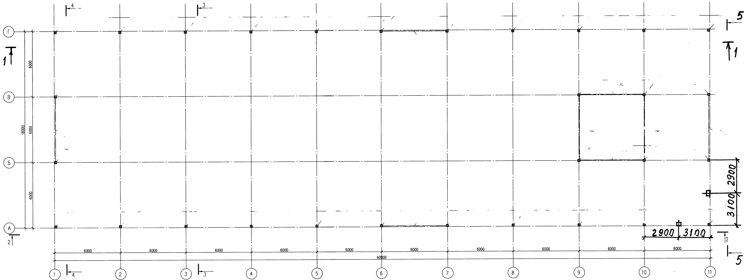
Схема расположения колонн
